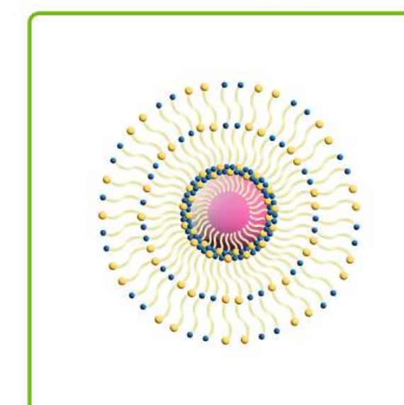
Схема строения капли масла с ламеллярной структурой
